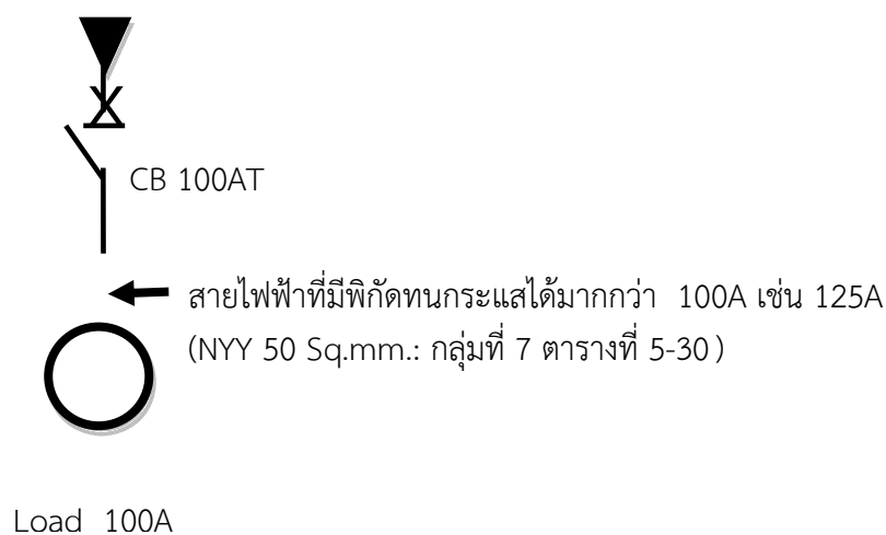
ภาพ วงจรและการเลือกใช้ใช้งานเซอร์กิตเบรกเกอร์
