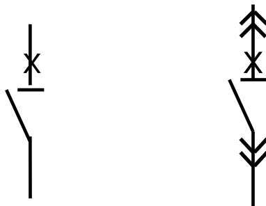
รูปที่ 1 ภาพสัญลักษณ์ของเซอร์กิตเบรกเกอร์ทั่วไป และเซอร์กิตเบรกเกอร์แบบ withdrawable ตามมาตรฐาน IEC ตามลำดับ
