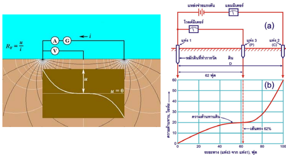
รูปที่ 5 แสดงการวัดค่าความต้านทานของระบบต่อลงดิน [14]
